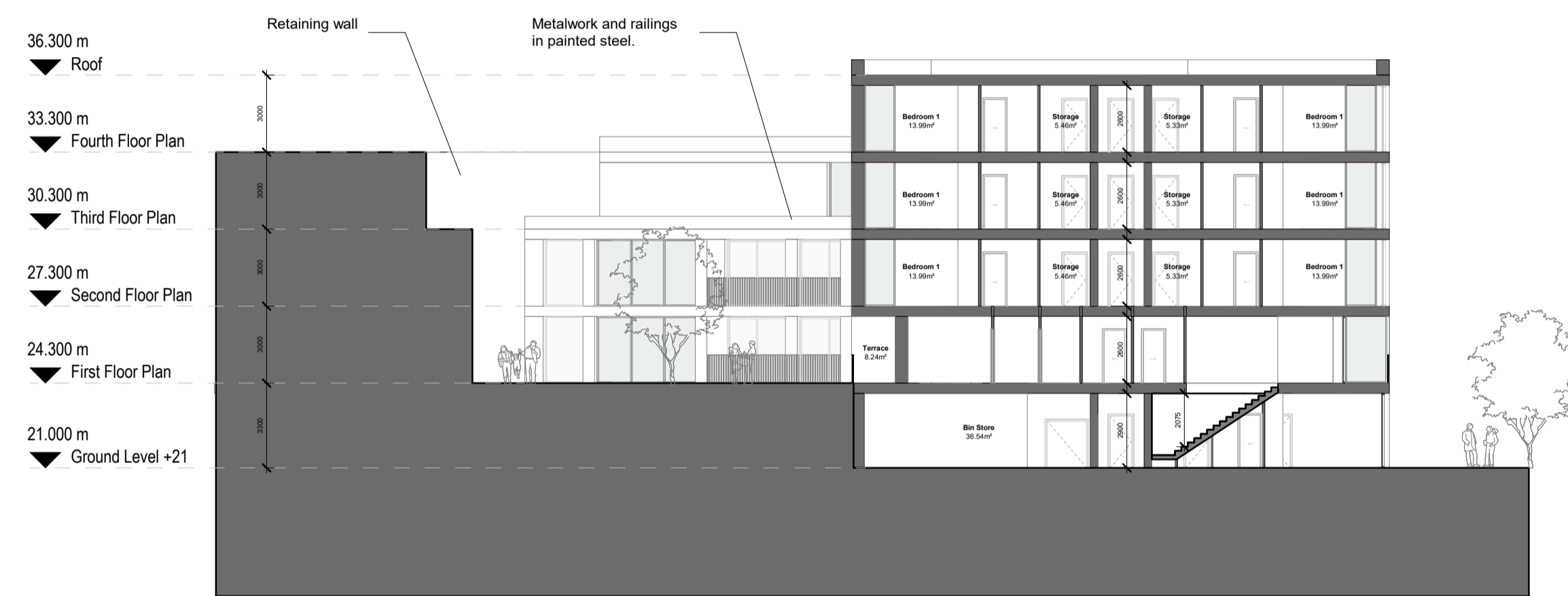
1 Section B-B 1 : 200
